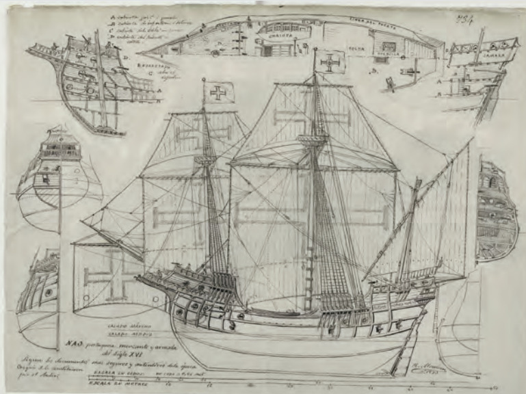
Estudio realizado por R. Monleón sobre el modelo de nao portuguesa del siglo XVI, seguido para construir parte de la flota para viajar a las islas de las especias en 1525.
